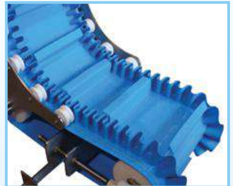
Băng tải SuperDrive TM chữ Z dán gờ cao, dẫn hướng và tai bèo
